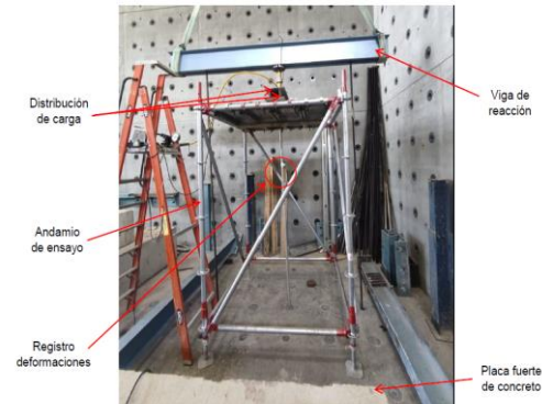
Foto No.13-1 Montaje del ensayo de servicio sobre andamio.
